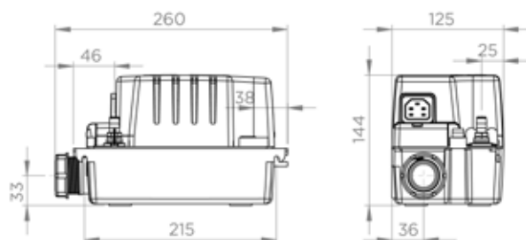
Afmetingen (mm)
